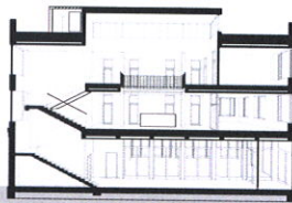
Řez podélný | M 1:200
