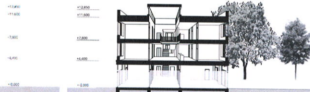
Řez příčný | M 1:200
