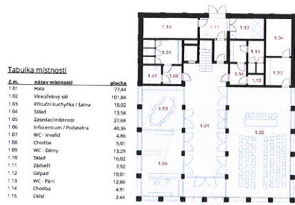
Půdorys 1.NP | M 1:200
